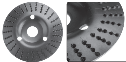
Abb. 10, Rapselscheibe
